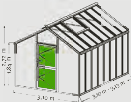
Bio-top III t-line mit 0,50 m Verglasungsraster
