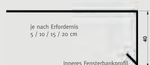
Inneres Fensterbankprofil
