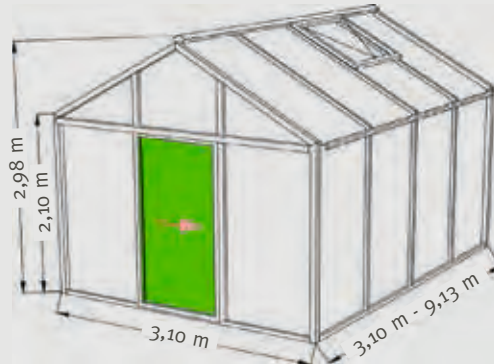
Bio-Varis L mit 1,00 m Verglasungsraster
