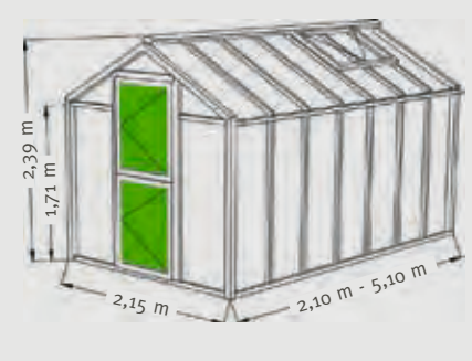
Bio-top I t-line mit 0,50 m Verglasungsraster
