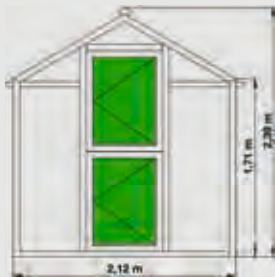
Standard: geteilte Drehtür Türbreite: ca. 0,73 m
