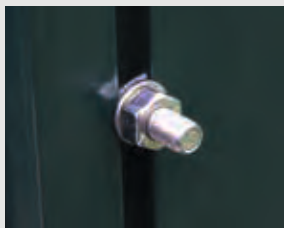
Hammerkopfschraube aus Edelstahl mit Mutter VE: 20 Stück, M6 x 16
