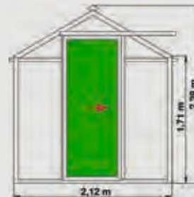
Alternativ: Schiebetür Türbreite: ca. 0,73 m
