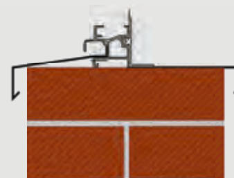
Abdeckung vom Mauerwerk mit Verbindungs- und Eckprofilen. Profile werden standardmäßig in der Farbe des Gewächshauses geliefert.
