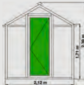
Alternativ: ungeteilte Drehtür Türbreite: ca. 0,73 m
