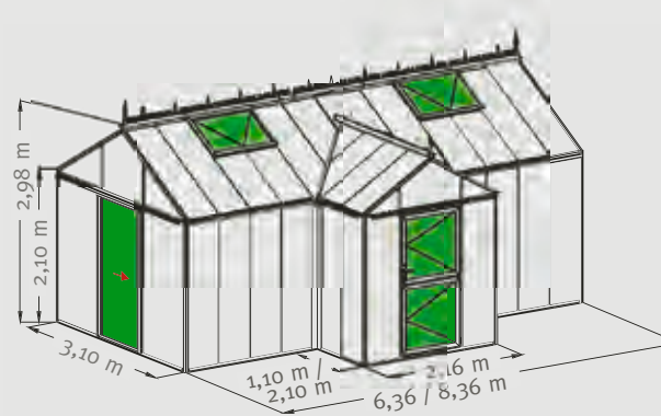
York t-line mit 0,50 m Verglasungsraster
