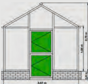
Standard: geteilte Drehtür Türbreite: ca. 0,93 m
