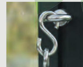
S-Haken (rostfrei) Größe: 27 x 49 mm VE: 10 Stück
