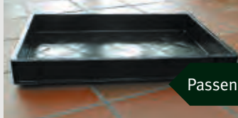
Transport- und Pflanzschale – besonders stabile Ausführung Farbe: schwarz, Inhalt: ca. 15 l, Maße: 60 x 40 x 9 cm
