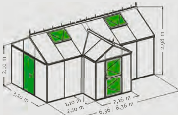
York mit 1,00 m Verglasungsraster
